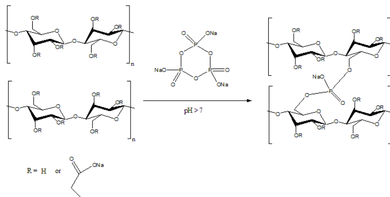
Рис. 8. Схема реакции КМЦ и триметафосфата натрия (ТМФ).
