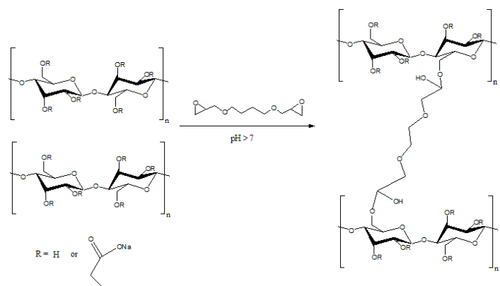
Рис. 5. Схема реакции КМЦ и 1,4-бутандиолдиглицилового эфира (БДДЭ).
