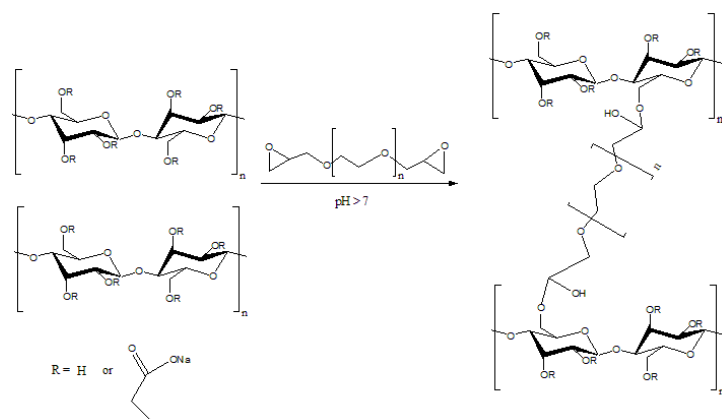
Рис. 6. Схема реакции КМЦ и полиэтиленгликольдиглицилового эфира (ПЭГДЭ).
