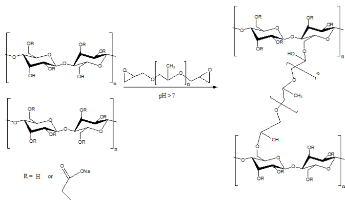
Рис. 7. Схема реакции КМЦ и полипропиленгликольдиглицилового эфира (ППГДЭ).
